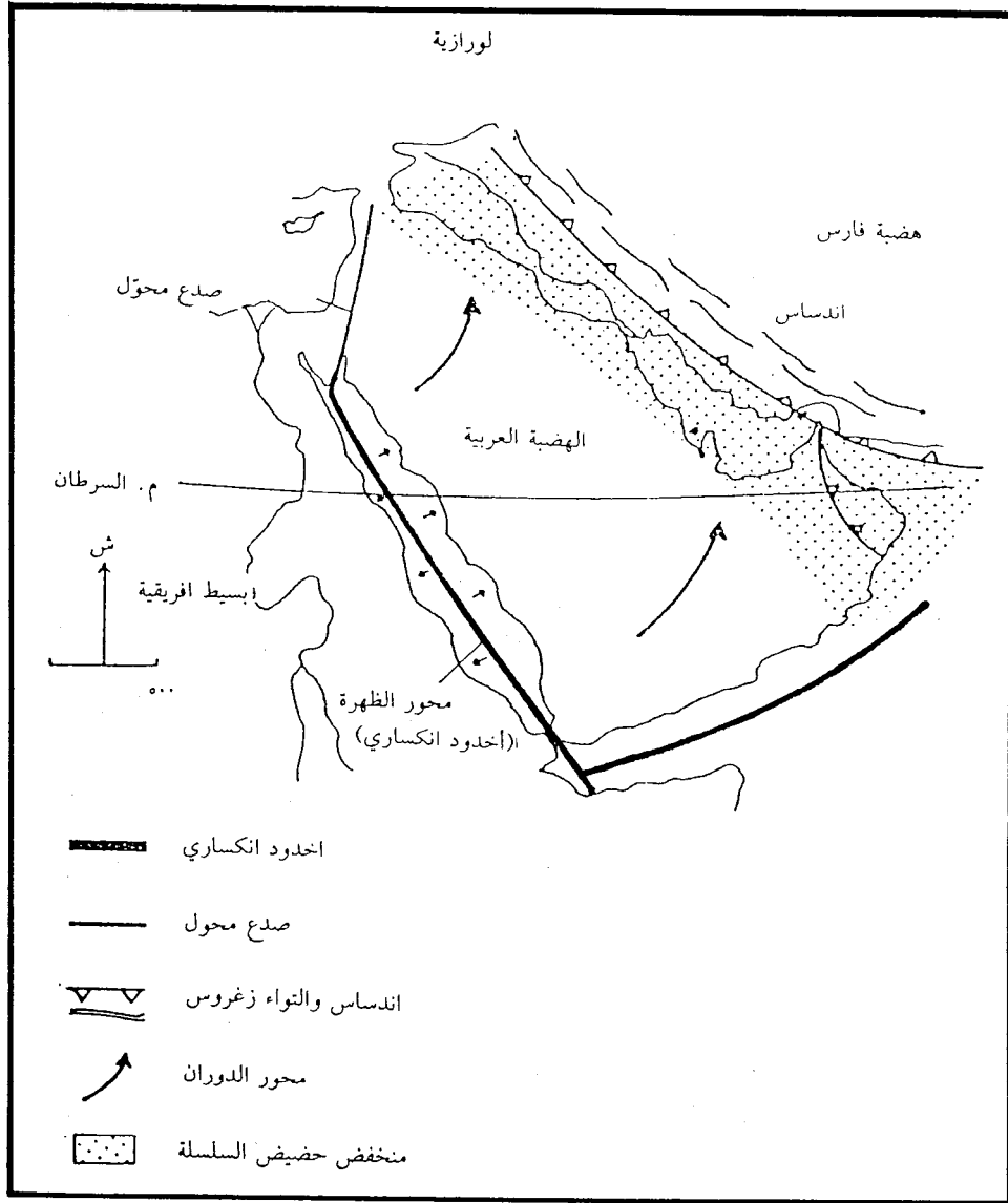
شكل ٢ - مخطط بنائي عام لتشكيل البحر الأحمر والخليج العربي
