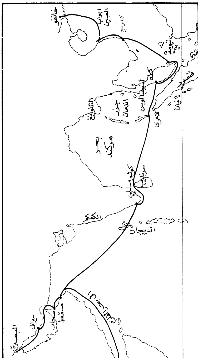
شكل ١٨ - الطريق البحرية من سيرا ف إلى خانقو
