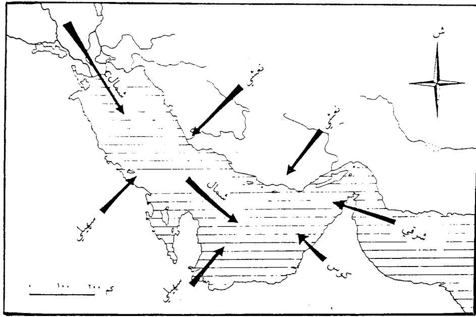
شكل ٥ - أنظمة الرياح الرئيسية في الخليج العربي
